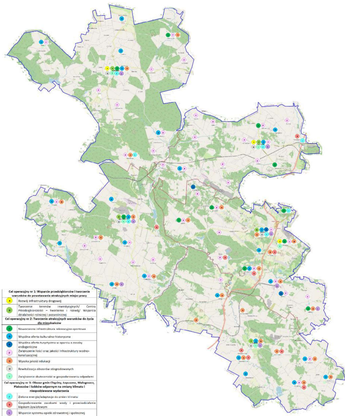
Mapa 18. Model struktury funkcjonalno-przestrzennej – działania źródło: opracowanie własne
