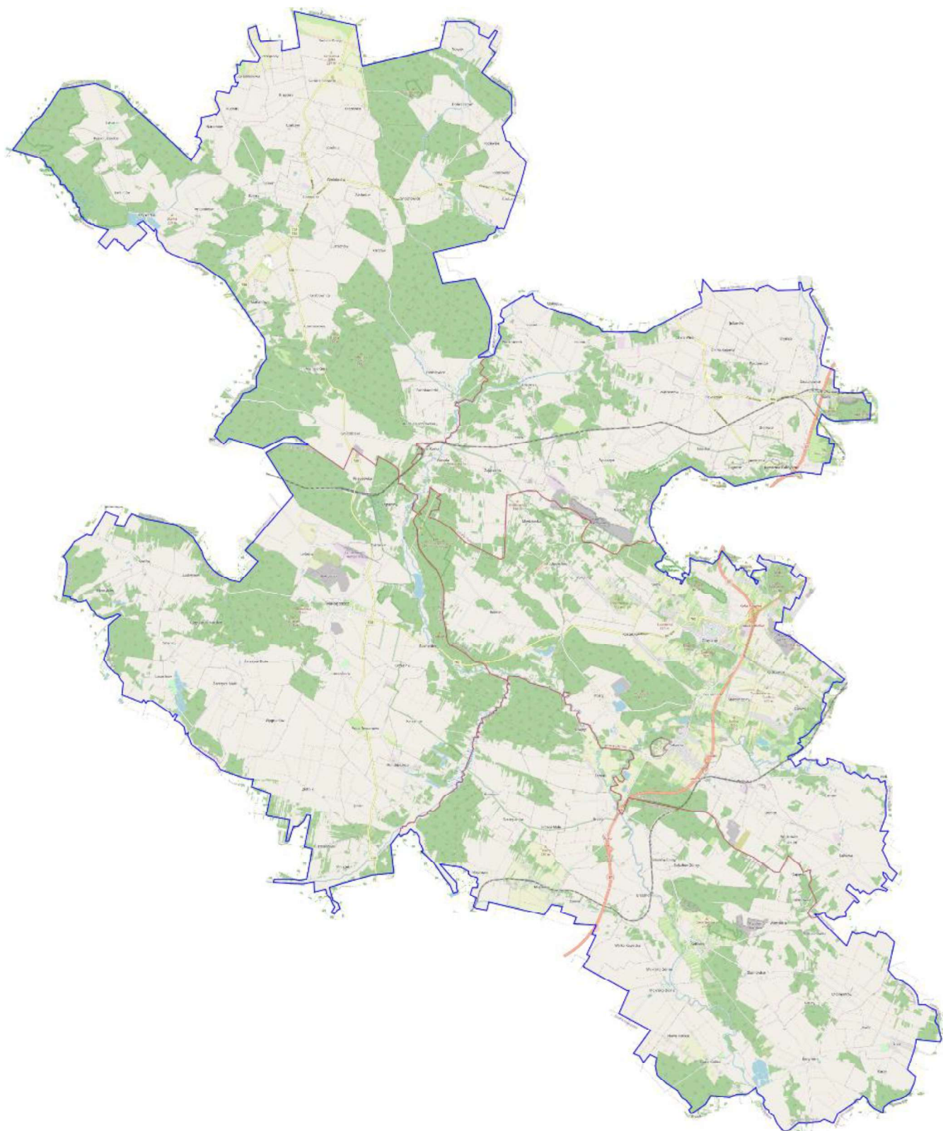
Mapa 13. Model struktury funkcjonalno-przestrzennej – komunikacja źródło: opracowanie własne
