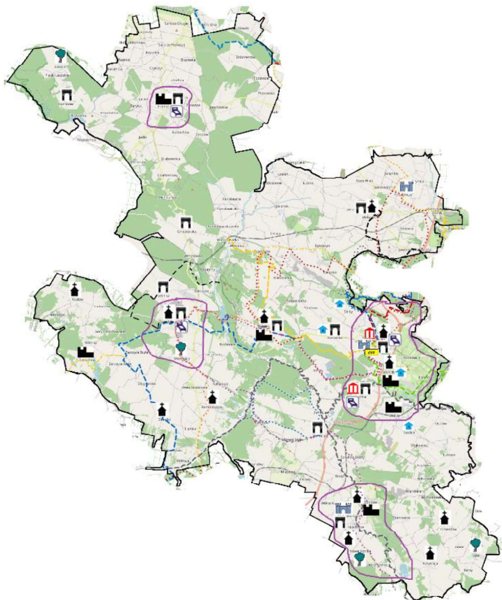
Mapa 15. Model struktury funkcjonalno-przestrzennej – turystyka źródło: opracowanie własne
